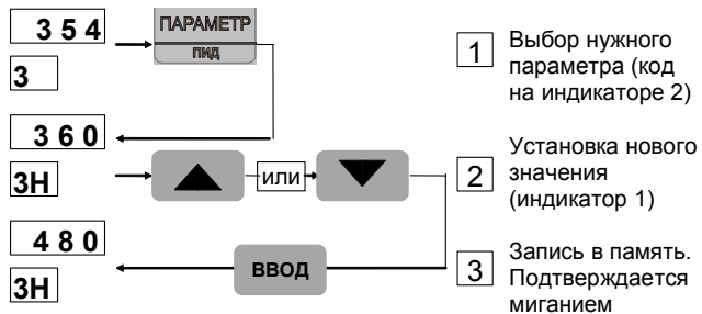
Рисунок 24 – Установка и просмотр параметров меню
