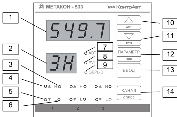
Рисунок 23 – Лицевая панель приборов «МЕТАКОН-533»
