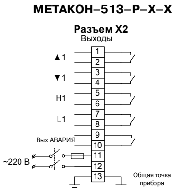
Рисунок 12 – Схема подключения выходных цепей к приборам модификации МЕТАКОН-513-P-X-X
