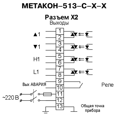
Рисунок 13 – Схема подключения выходных цепей к приборам модификации МЕТАКОН-513-C-X-X
