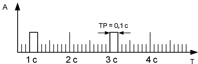
Рисунок 5 – Диаграммы работы ШИМ-модулятора без ограничения минимальной длительности импульса и с ограничением.
