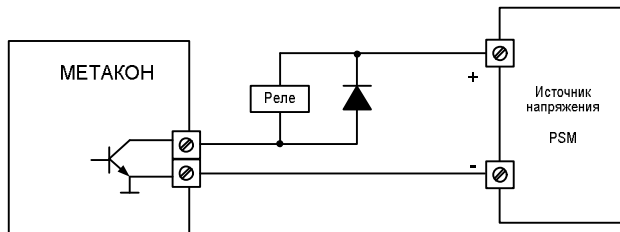
Рисунок 21 – Схема подключения электромеханического реле постоянного напряжения к выходу типа «Т»
