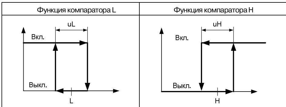
Рисунок 6 – Функции компараторов Н и L.
