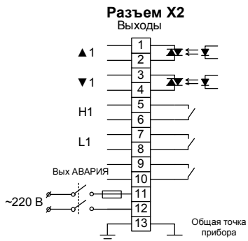
Рисунок 14 – Схема подключения выходных цепей к приборам модификаций МЕТАКОН-513-CP-X-X
