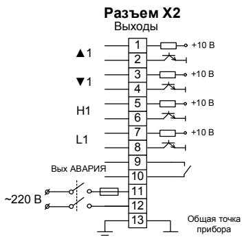
Рисунок 15 – Схема подключения выходных цепей к приборам модификаций МЕТАКОН-513-K-X-X
