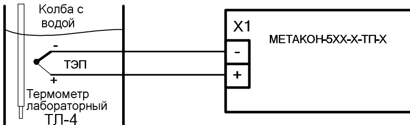
Рисунок А.6.3.1.2 – Схема подключения приборов МЕТАКОН 5ХХ-Х-ТП-Х для поверки погрешности компенсации влияния температуры холодных спаев.
