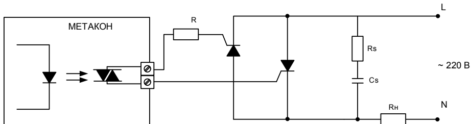
Рисунок 20 – Схема подключения силовых тиристоров к выходу типа «С» 4.5.3 Подключение нагрузки к транзисторному выходу типа «Т»
