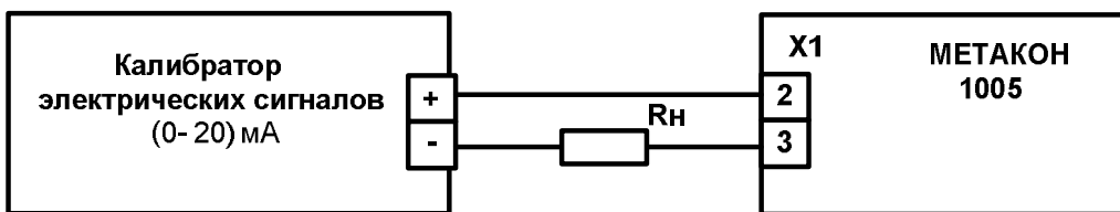
Рисунок А.6.3.1.2 – Схема подключения прибора МЕТАКОН-1005 для проведения проверки по сигналам тока
