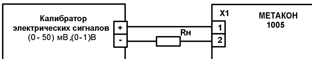
Рисунок А.6.3.1.1 – Схема подключения прибора МЕТАКОН-1005 для проведения проверки по сигналам напряжения
