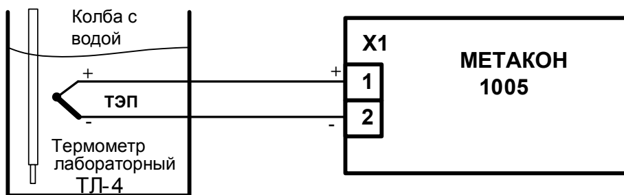
Рисунок А.6.3.2 – Схема проверки погрешности компенсации температуры холодного спая
