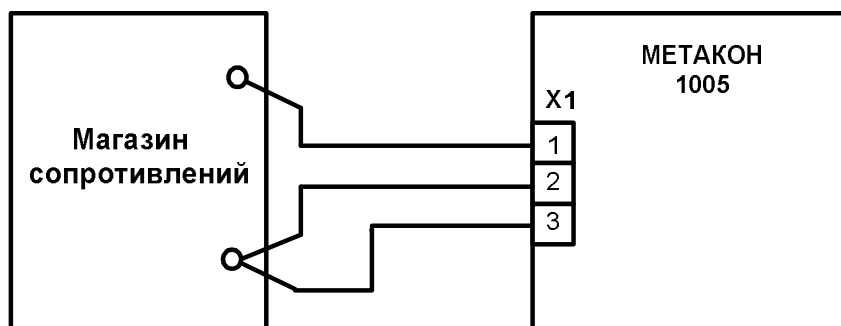
Рисунок А.6.3.1.3 – Схема подключения прибора МЕТАКОН-1005 для проведения проверки по сигналам сопротивления
