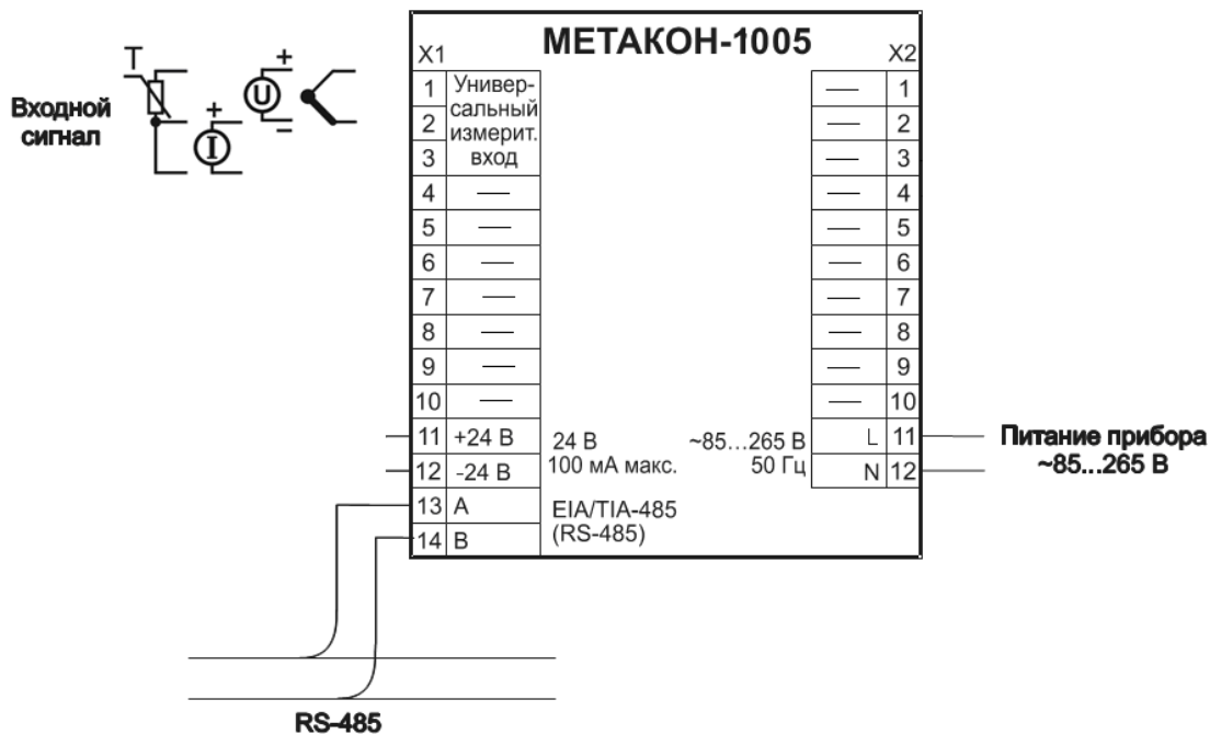
Рисунок 10 – Электрическая схема подключения прибора METAKON-1005
