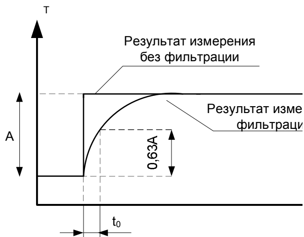
Рисунок 3 – График, показывающий влияние цифровой фильтрации результата измерения
