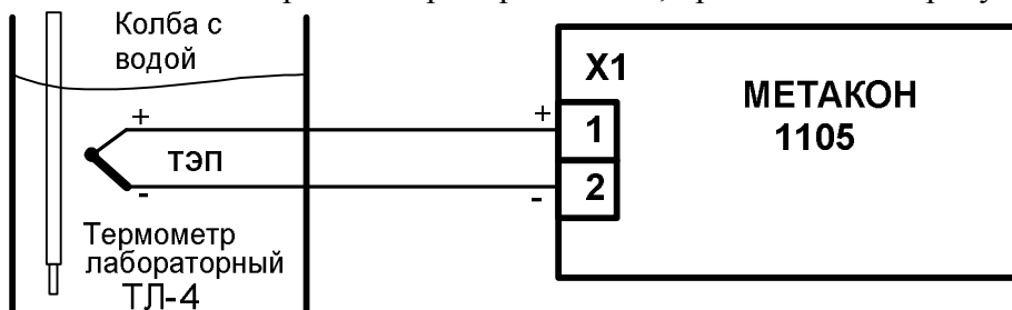
Рисунок А.6.3.2 – Схема проверки погрешности компенсации температуры холодного спая
