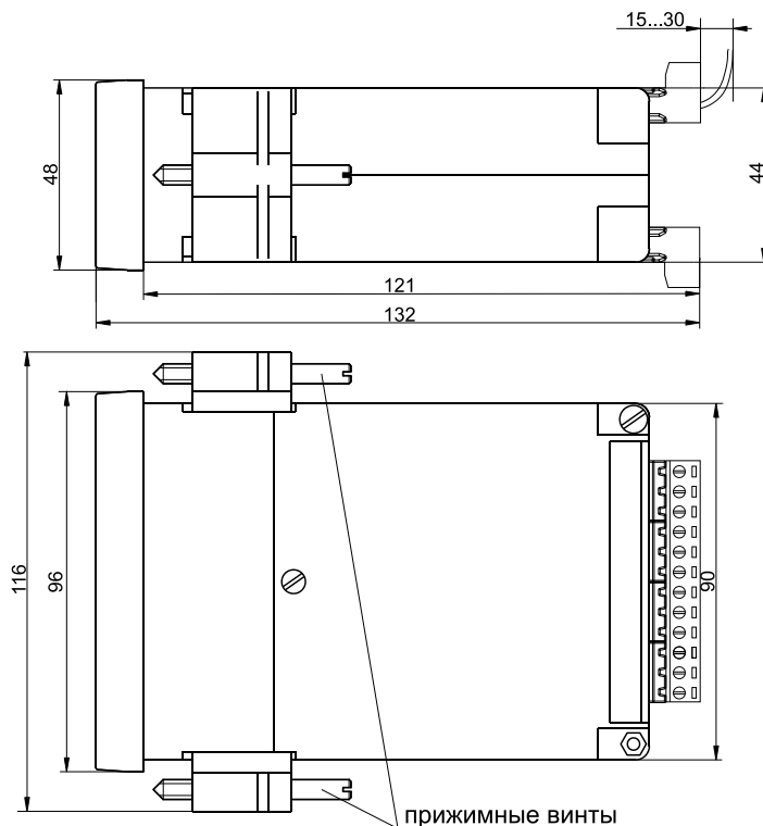
Рисунок 8 – Габаритные размеры прибора МЕТАКОН-1105
