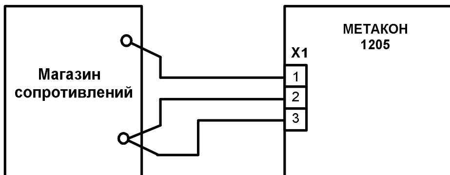
Рисунок А.6.3.1.3 – Схема подключения прибора МЕТАКОН-1205 для проведения проверки по сигналам сопротивления
