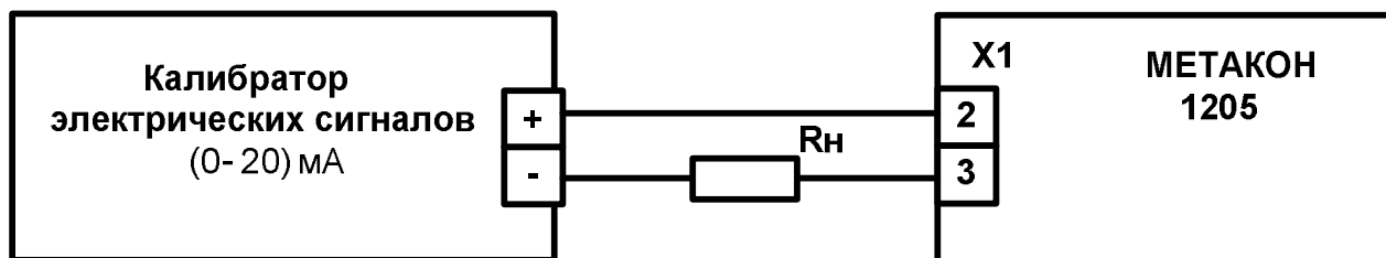
Рисунок А.6.3.1.2 – Схема подключения прибора МЕТАКОН-1205 для проведения проверки по сигналам тока
