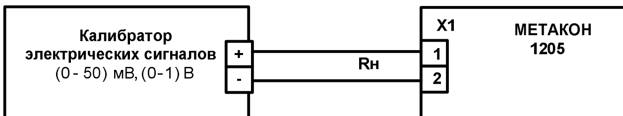
Рисунок А.6.3.1.1 – Схема подключения прибора МЕТАКОН-1205 для проведения проверки по сигналам напряжения
