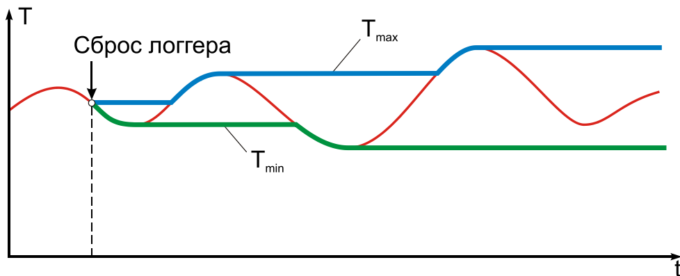
Рисунок 7 – Функция логгера прибора
