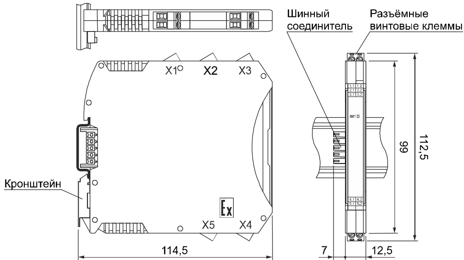
Рисунок 6.1 – Габаритные размеры барьера КА5011Ex-NN
