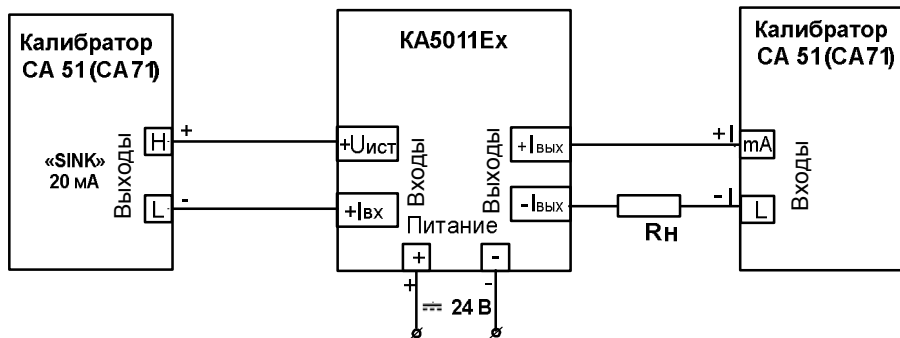
Рисунок 6.4.1А – Подключение барьеров мод. KA5011Ex для проверки преобразования входных унифицированных сигналов постоянного тока (входной пассивный сигнал) в диапазоне от 4 до 20 мА в выходной унифицированный сигнал постоянного тока от 4 до 20 мА
