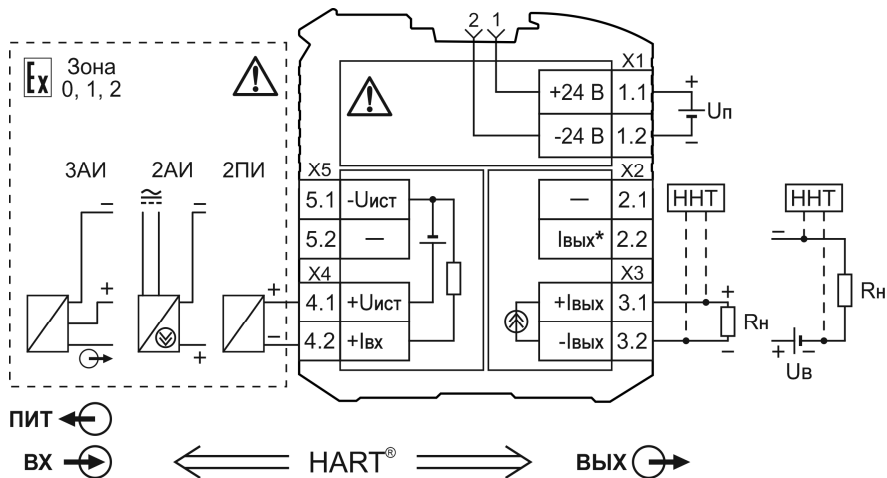
Рисунок 6.2 – Типовые схемы подключения барьеров KA5011Ex-NN
