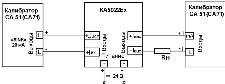
Рисунок 6.4.1А – Подключение барьеров мод. KA5022Ex для проверки преобразования входных унифицированных сигналов постоянного тока (входной пассивный сигнал) в диапазоне от 4 до 20 мА в выходной унифицированный сигнал постоянного тока от 4 до 20 мА
