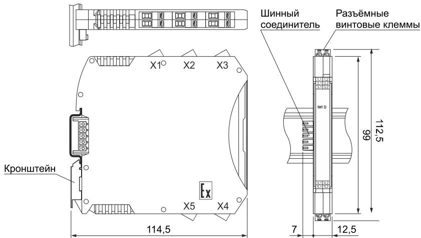
Рисунок 6.1 – Габаритные размеры барьера KA5022Ex-10
