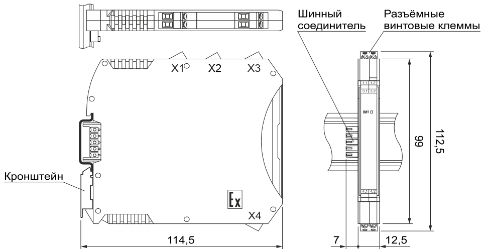
Рисунок 6.1 – Габаритные размеры барьера KA5031Ex-1N
