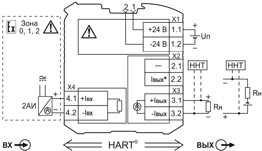
Рисунок 6.2 – Типовая схема подключения барьеров KA5031Ex-1N
