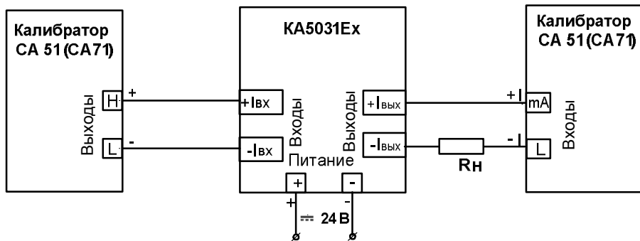
Рисунок 6.4.1А – Подключение барьеров мод. KA5031Ех для проверки преобразования входных унифицированных сигналов постоянного тока (входной пассивный сигнал) в диапазоне от 4 до 20 мА в выходной унифицированный сигнал постоянного тока от 4 до 20 мА
