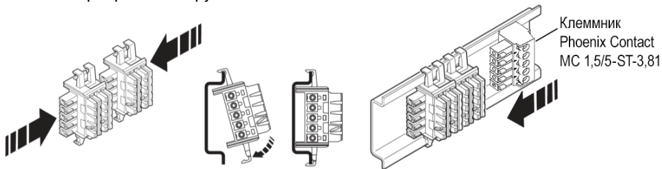
Рисунок 6.3 – Установка шинных соединителей на DIN-рейку, а также место установки клеммного соединителя Phoenix Contact MC1,5/5-ST-3,81
