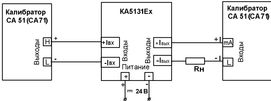
Рисунок 6.4.1А – Подключение барьеров мод. KA5131Ex для проверки преобразования входных унифицированных сигналов постоянного тока (входной пассивный сигнал) в диапазон от 4 до 20 мА в выходной унифицированный сигнал постоянного тока от 4 до 20 мА
