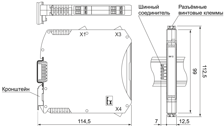
Рисунок 6.1 – Габаритные размеры барьера KA5131Ex-NN
